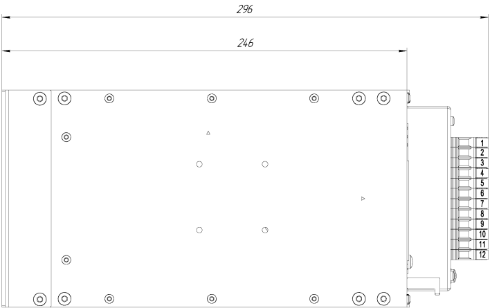
Рисунок Ж.2 – Габариты и установочные размеры устройства в исполнении «ЮНИТ-М314»
