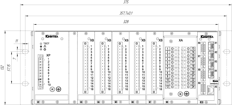
Рисунок Ж.2 – Габариты и установочные размеры устройства в исполнении «ЮНИТ-М314»
